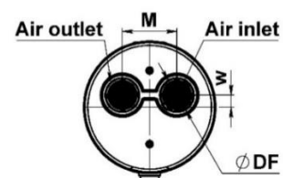
Εικ. 7 – Διαστάσεις
