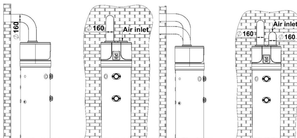
SI. 5a – Primer izhodnega prezračevalnega kanala SI. 5b – Primer dvojnega prezračevalnega kanala
