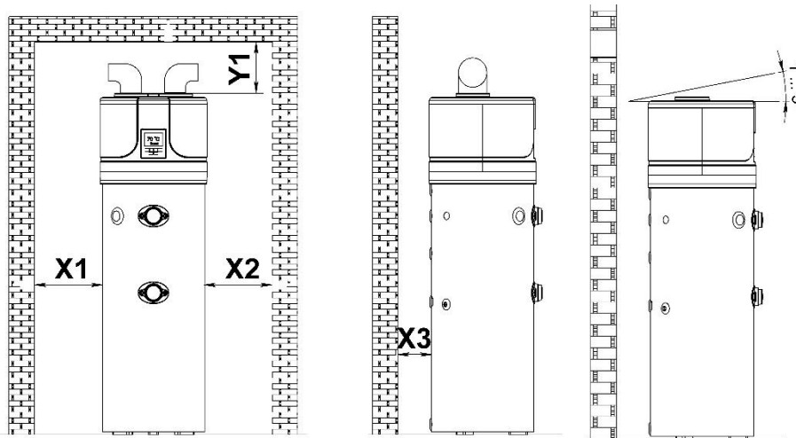
Sl. 4a – Minimalni prostor i ugradnja bez zračnih kanala.
