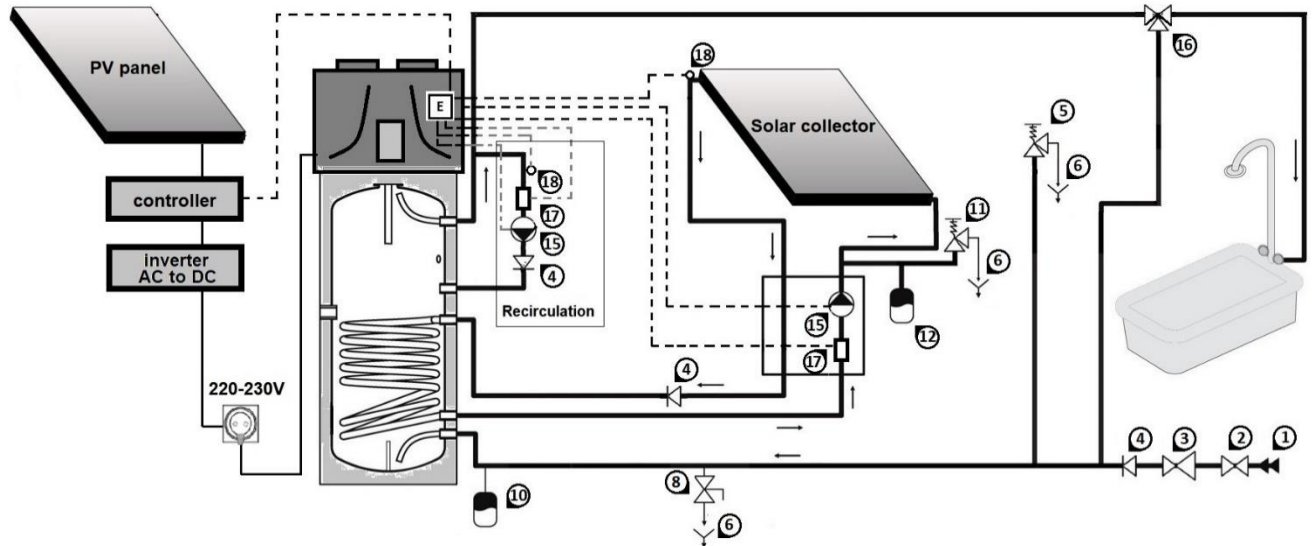
Εικ. 8 Σύνδεση με το σύστημα παροχής νερού και τον ηλιακό συλλέκτη
