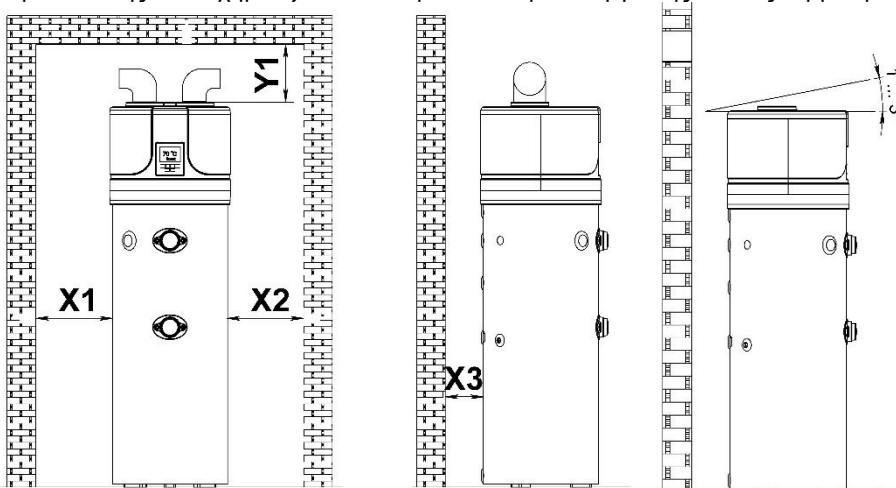
Εικ. 4a – Ελάχιστος χώρος και εγκατάσταση χωρίς αεραγωγούς.
