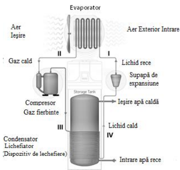
Fig.1 – Principiul de funcționare ►
