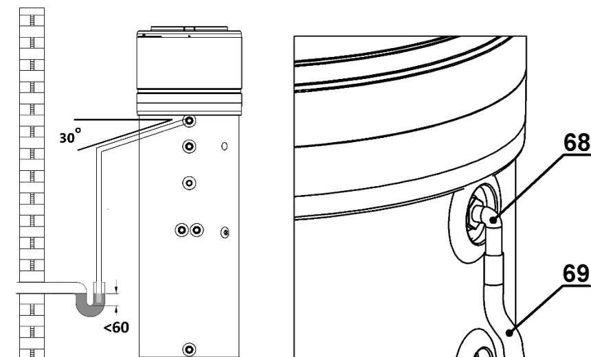
SI. 9 – Primjer povezivanja cijevi za odvod kondenzata putem sifona
