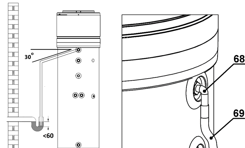
Sl.9–Primer povezivanja cevi za odvod kondenzata pomoću sifona
