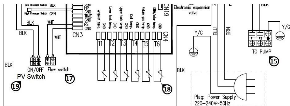
Εικ. 13. Καλωδίωση εξωτερικών συσκευών
