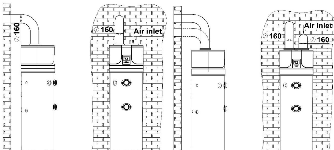
Sl. 5a – Primjer za izlazni zrakovod
