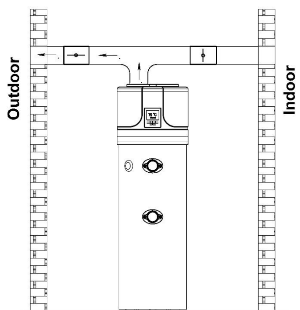
SI.6b Primer instalacije tokom zime
