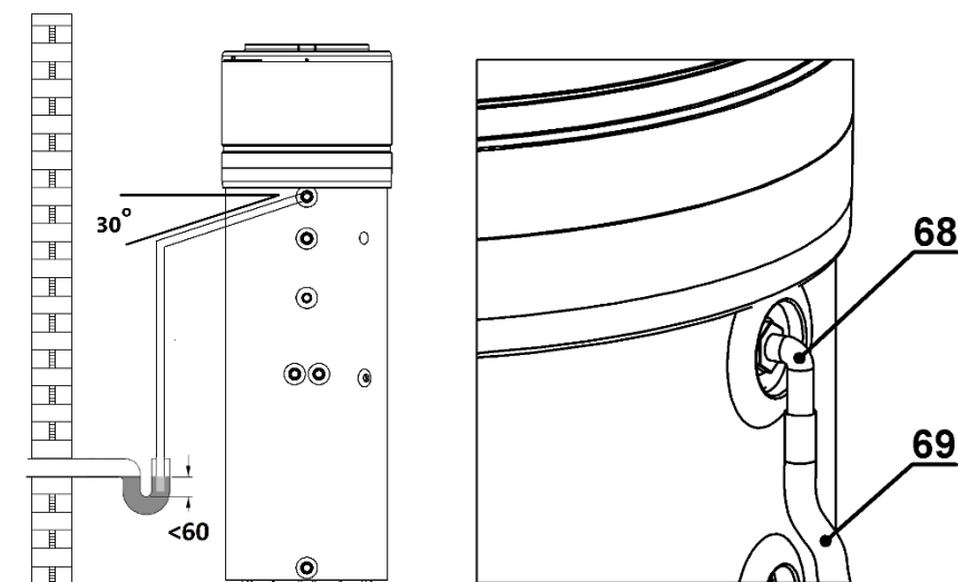
Фиг. 9 – Пример за свързване на отводнителната тръба на конденза чрез сифон
