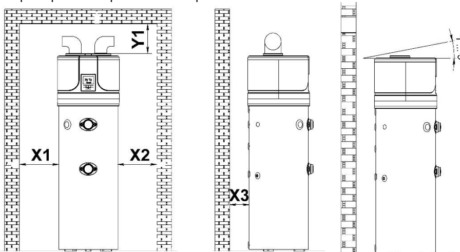
Фиг. 4а – Минимално пространство и инсталиране без въздуховоди.
