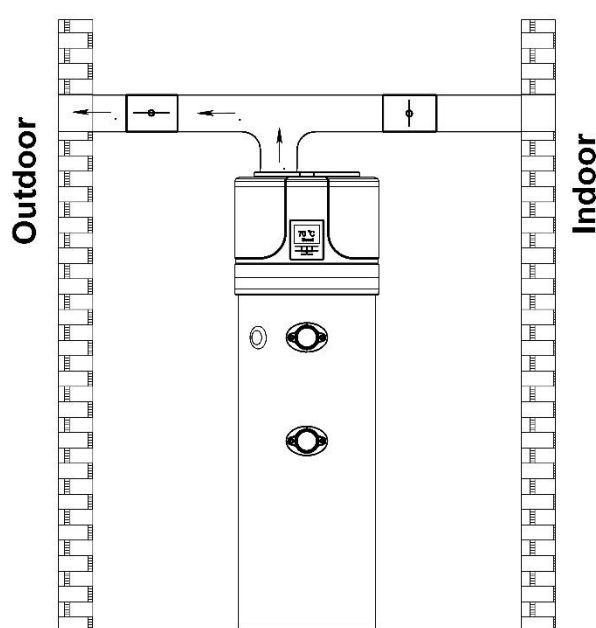
Фиг.6б Примерна инсталация през зимата
