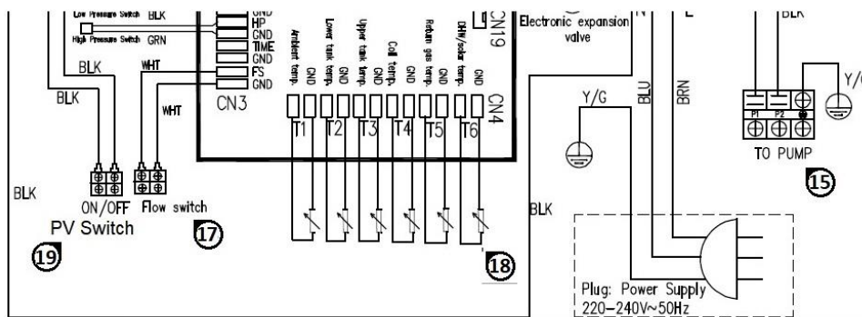
Sl. 13. Ožičenje spoljašnjih uređaja
