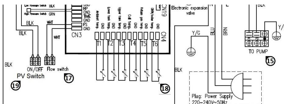
Fig. 13. Cablarea dispozitivelor externe
