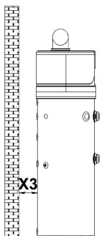
Fig. 4a – Spațiu minim și instalare fără conducte de aer
