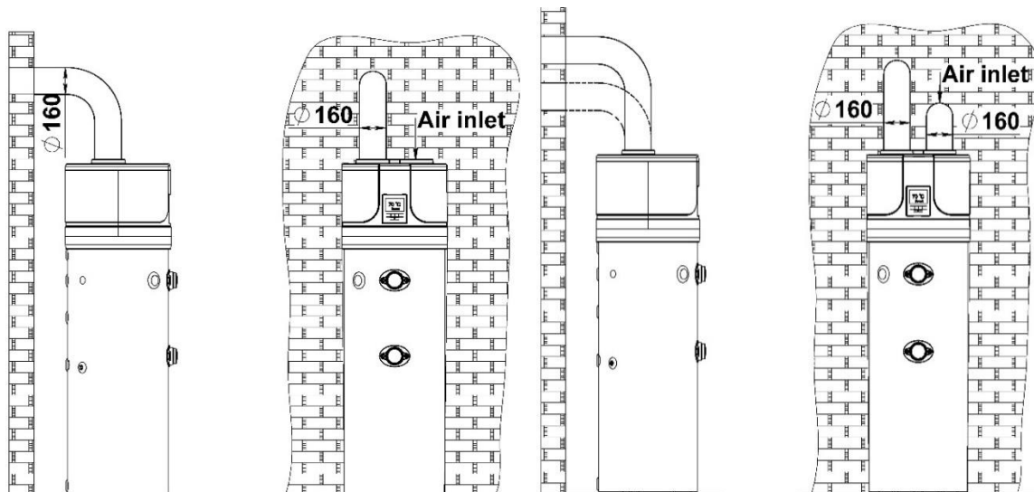
Εικ. 5a – Παράδειγμα αγωγού εξαγωγής
