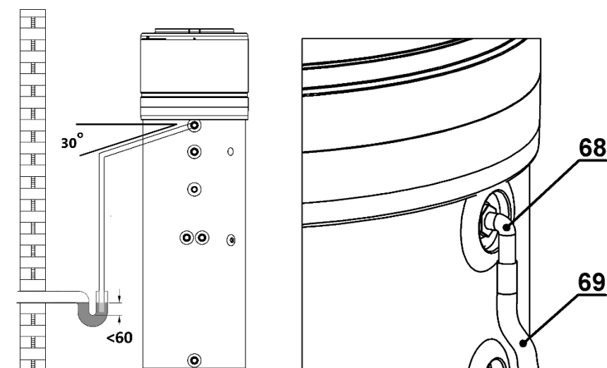
Sl. 9 – Primer povezave odtočne cevi za vlago preko sifona
