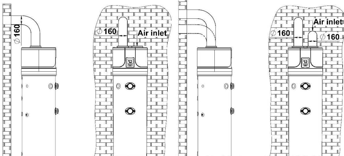
Sl. 5a – Primer za izlazni odvod vazduha
