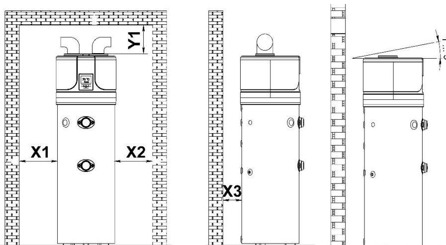
SI. 4a – Minimalne razdalje in montiranje brez prezračevalnih kanalov
