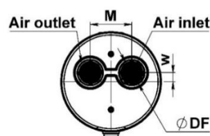
SI. 7 – Ukupne dimenzije
