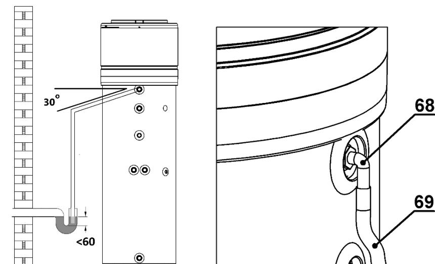
Εικ. 9 – Παράδειγμα σύνδεσης του σωλήνα αποστράγγισης συμπυκνωμάτων μέσω σιφόν
