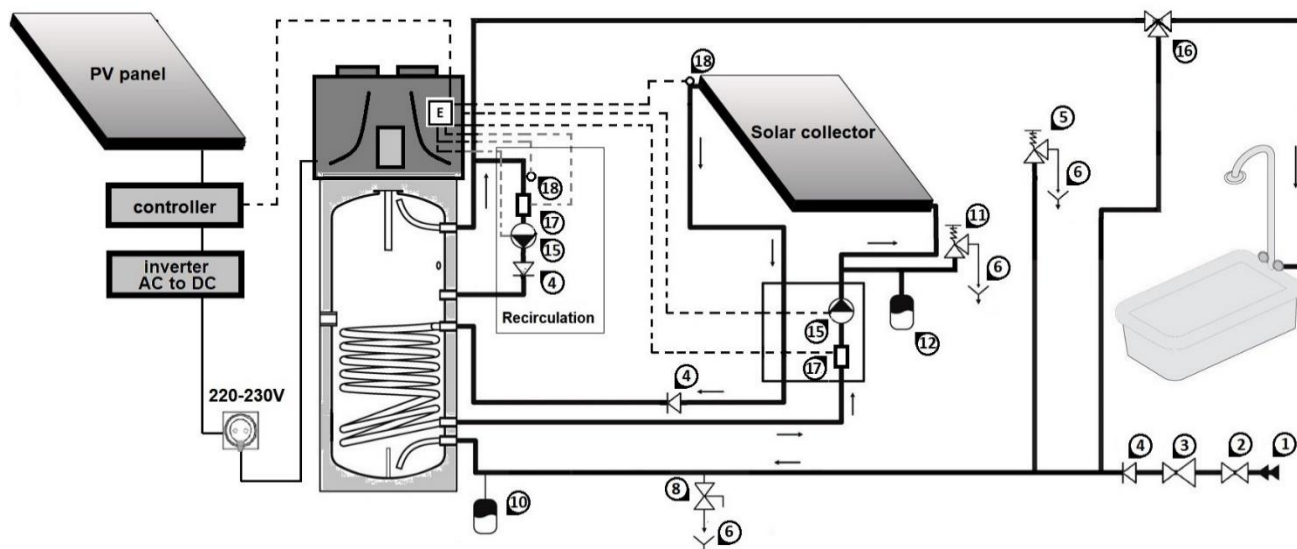
SI. 8 Priključak na sistem za snabdevanje vodom i solarni kolektor
