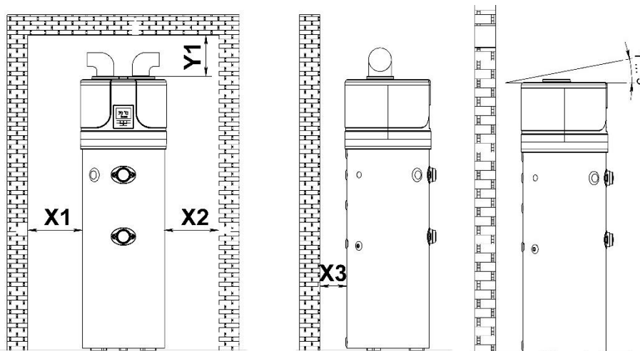
Sl.4a–Minimalni prostor i ugradnja bez vazdušnih kanala.
