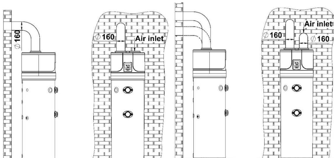
Фиг. 5а – Пример за отвеждащ въздуховод
