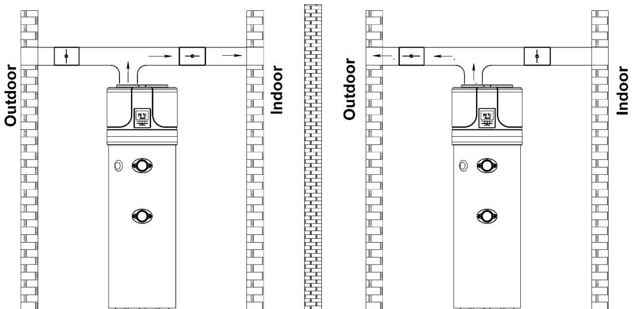
Εικ.6α – Παράδειγμα εγκατάστασης το καλοκαίρι Εικ.6β Παράδειγμα εγκατάστασης το χειμώνα
