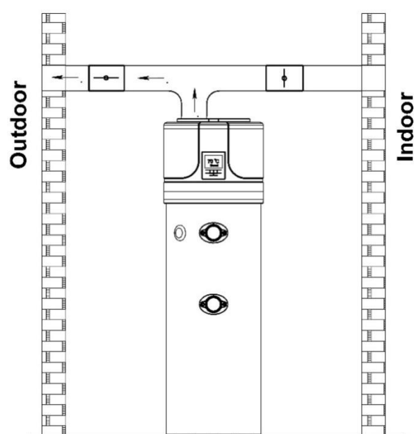
Sl. 6b Primer instalacije pozimi
